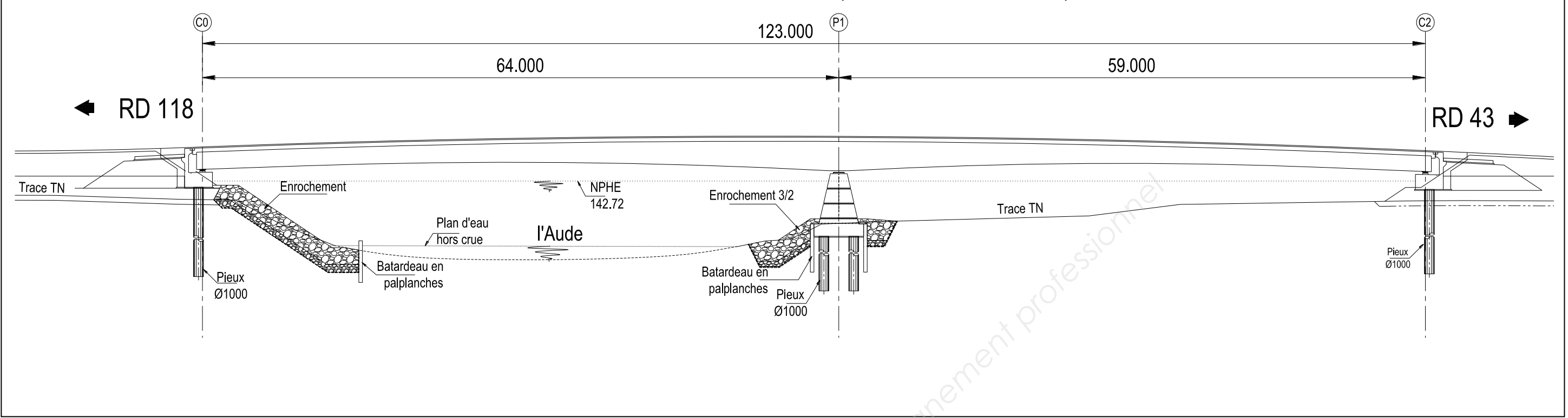
COUPE TRANSVERSALE DU TABLIER (sans indication d'échelle)
