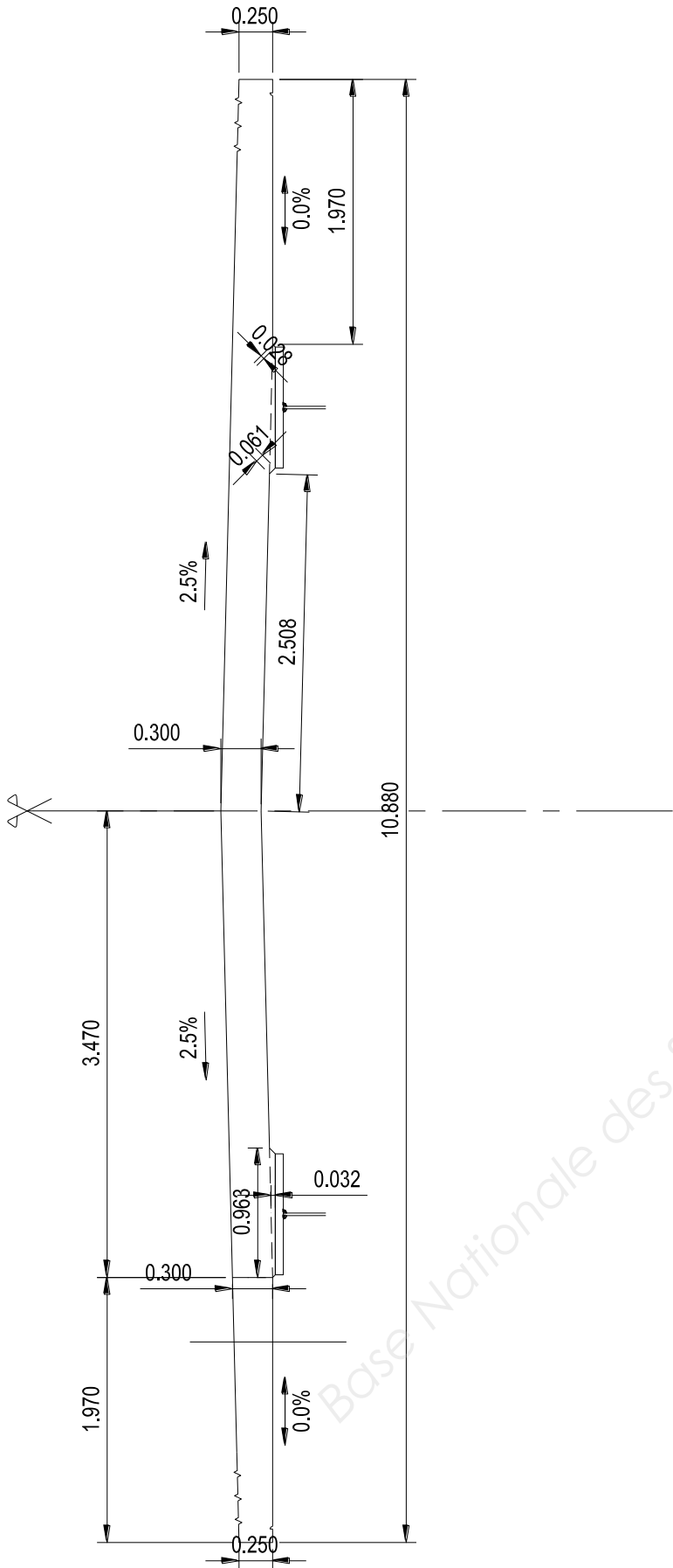
COUPE TRANSVERSALE DU HOURDIS
